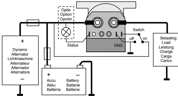
Aansluitschema voor een op afstand bediende hoofdschakelaar Connection diagram for a remote operated main switch
